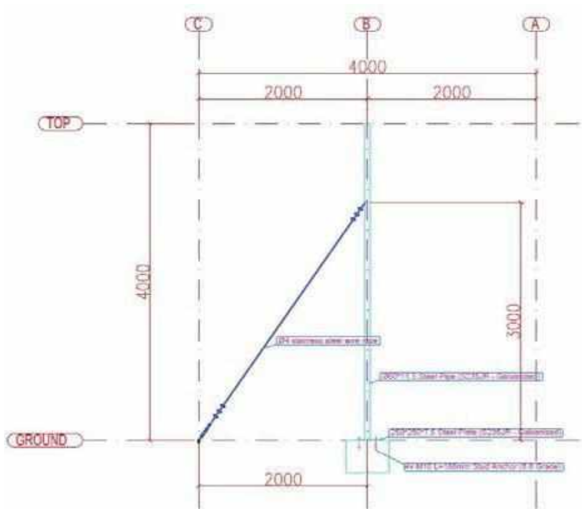
Рисунок 8 – Схема крепления
