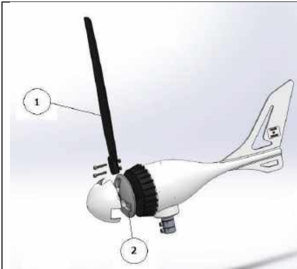
Рисунок 5 – Сборка ветрогенератора.
