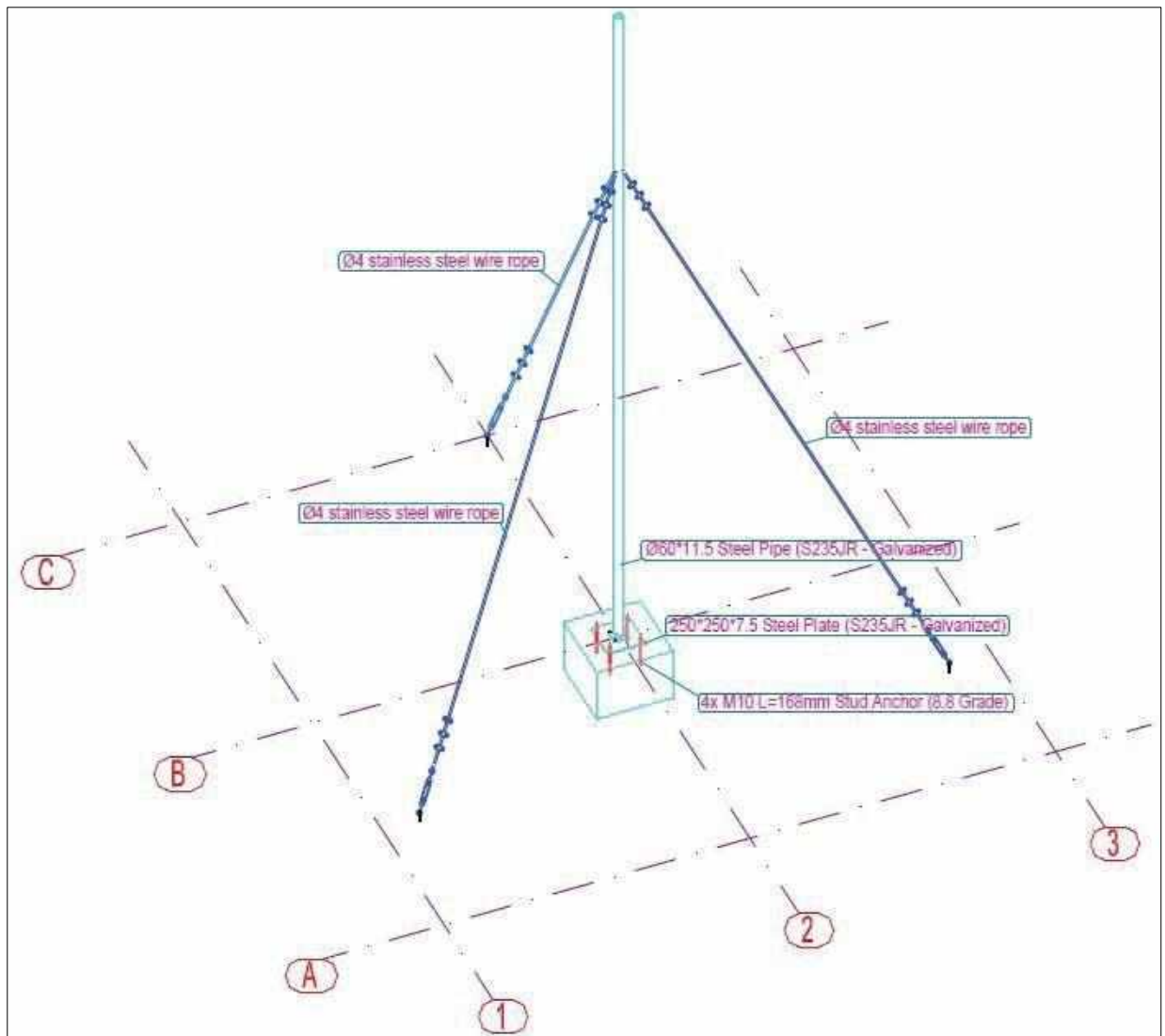
Рисунок 7 – Схема основания для установки мачты.
