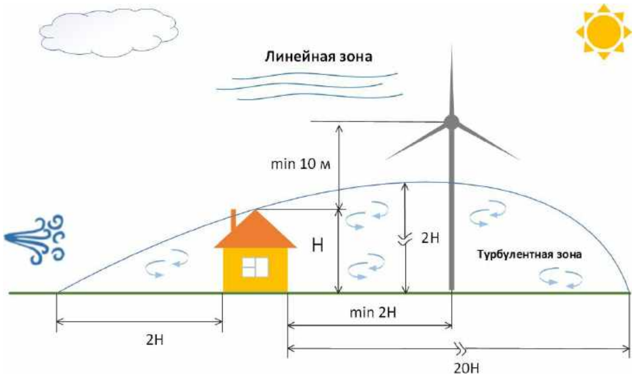
Рисунок 3 – Расположение ветрогенератора по отношению к препятствиям.
