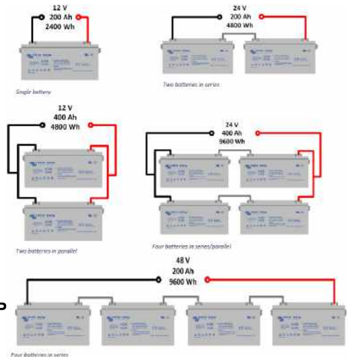
Рисунок 8 – Схемы подключения аккумуляторных батарей.
