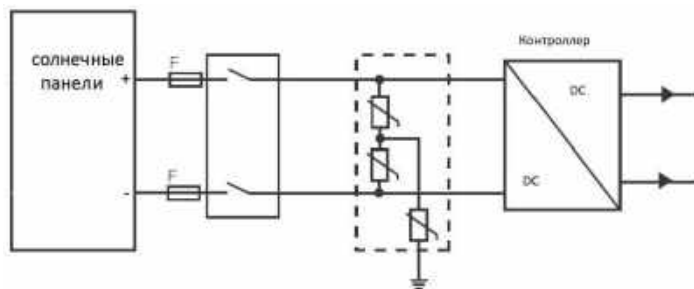
Рисунок 7 Принципиальная схема установки предохранителей и УЗИП в линию постоянного тока
