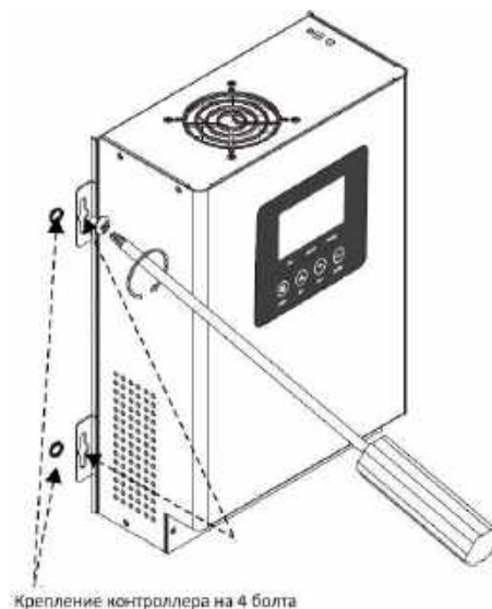
Рисунок 5 Крепление на стену
