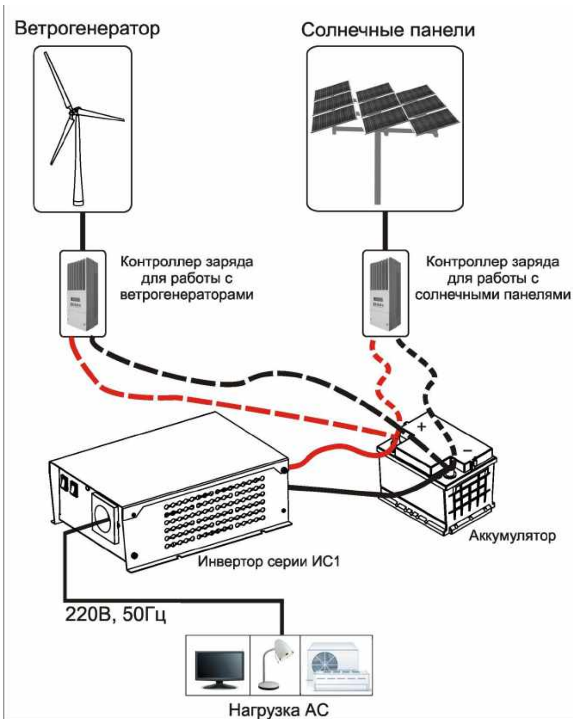
Рис.7. Схема подключения инверторов серии ИС1-XX-XXXX P к системам альтернативной энергетики
