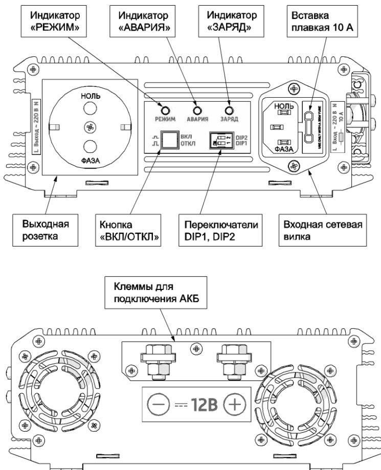
Рис.4. Панели СибРезерв 1000
