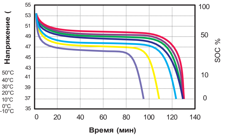
Разряд при различной температуре
