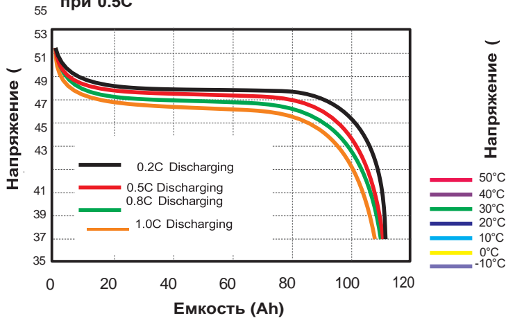
Графики разряда разными токами при 25°C при 0.5C
